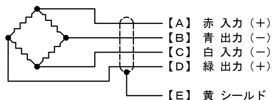
4 芯ケーブル接続図
